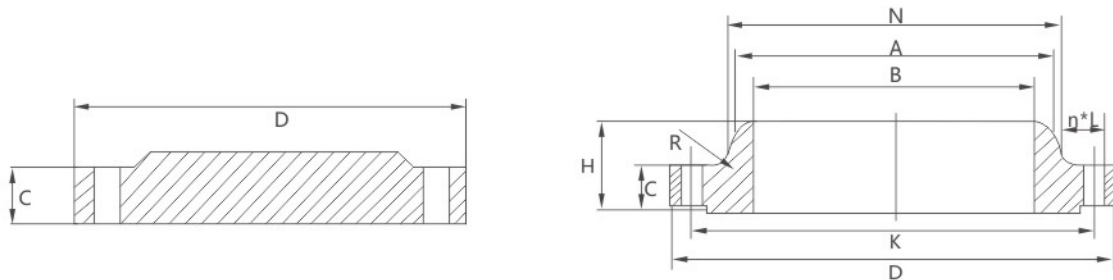
Class300(PN50) A系列大直径钢制管法兰和法兰盖
